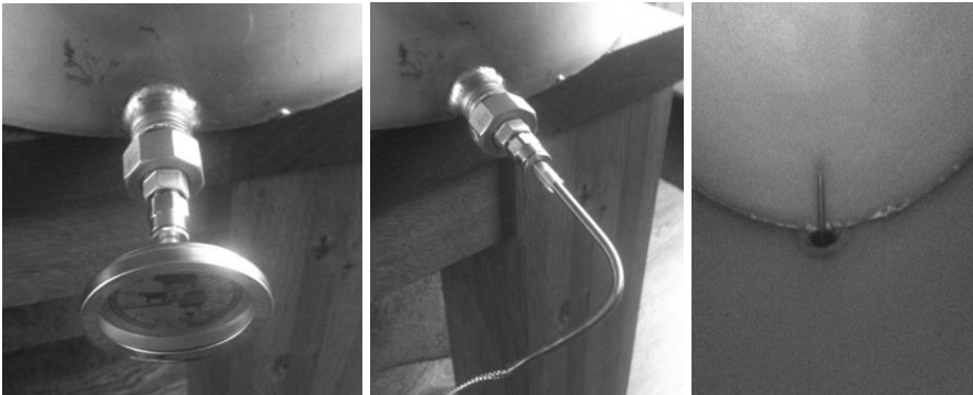
Braad thermometer in pan gemonteerd + binnen aanzicht in pan
